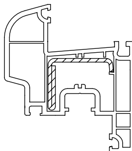
Армирование 35 x 28
