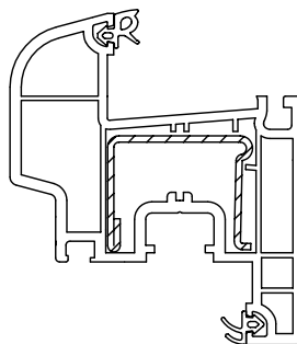
Уплотнитель притвора
