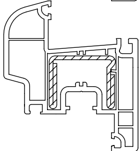
Армирование 35 x 28
