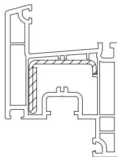
Армирование 35 x 28
