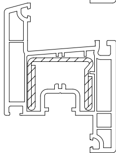
Армирование 35 x 28
